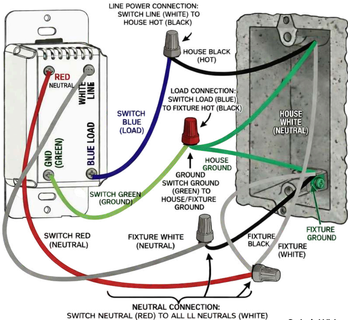
Switch Wiring
